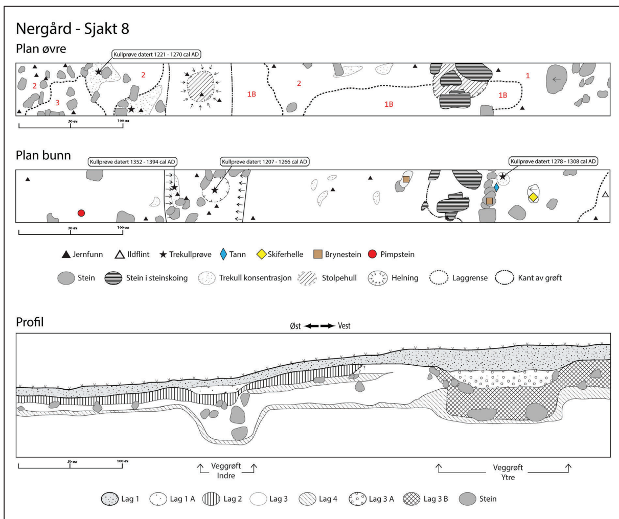
Figur 4. Sjakt 8 profiltegning mot sør og plantegninger fra øvre del og bunn av sjakta i tuft 2. Illustrasjon: Stephen Wickler og Jon Gunnar Blom, UM
