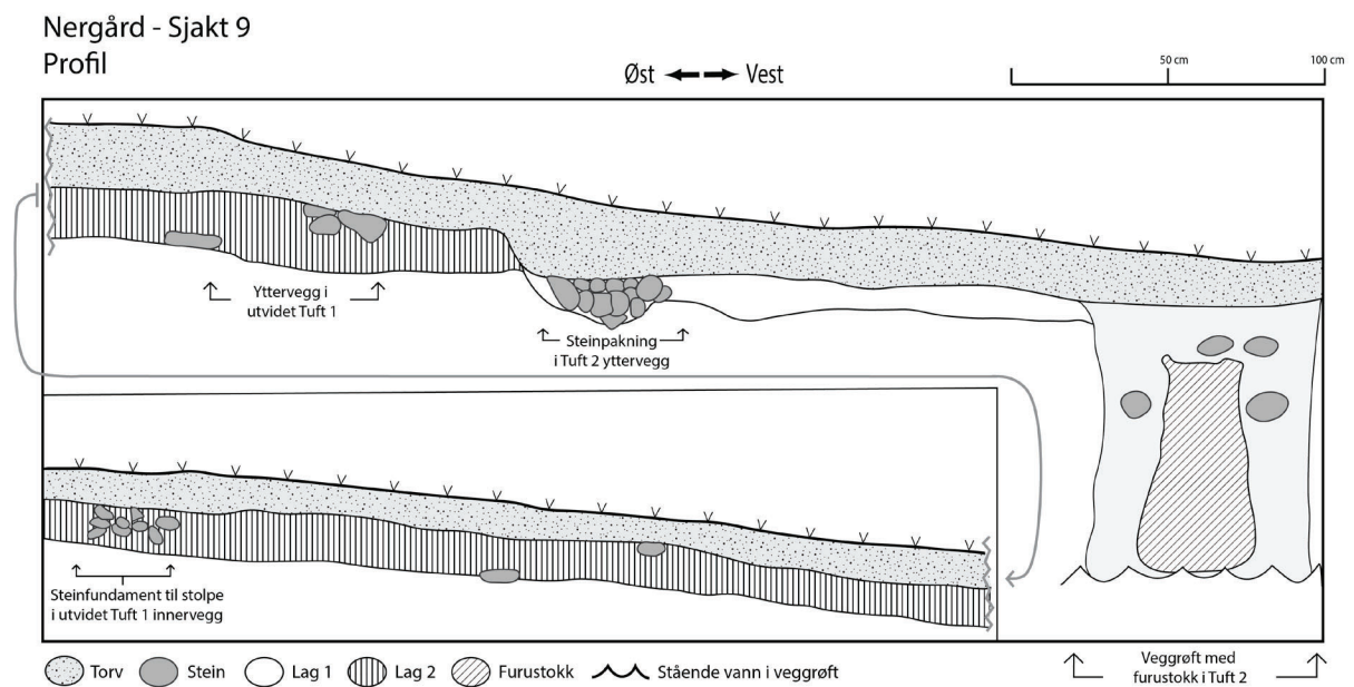
Figur 21. Sjakt 9 profiltegning mot sør. Illustrasjon: TFFK og Jon Gunnar Blom, UM
